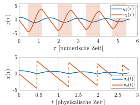
Abbildung 3. Trajektorien als Funktion der numerischen Zeit (oben), die roten Streifen markieren Intervalle, in denen die Hilfsdynamik aktiv war. Verlauf der rekonstruierten un stetigen Trajektorien als Funktion der physikalischen Zeit (unten).
